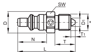
Ниппель без клапана (проходного типа) / Through type adaptor (without valve) HP-004-1-XX002-12-Y13
