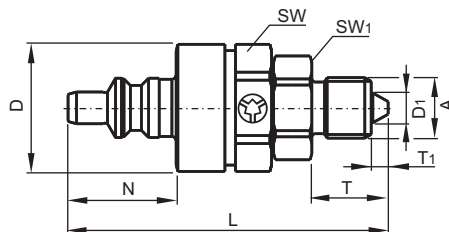
Ниппель с клапаном / Self sealing adaptor (with valve) HP-004-2-XX002-12-2-Y13
